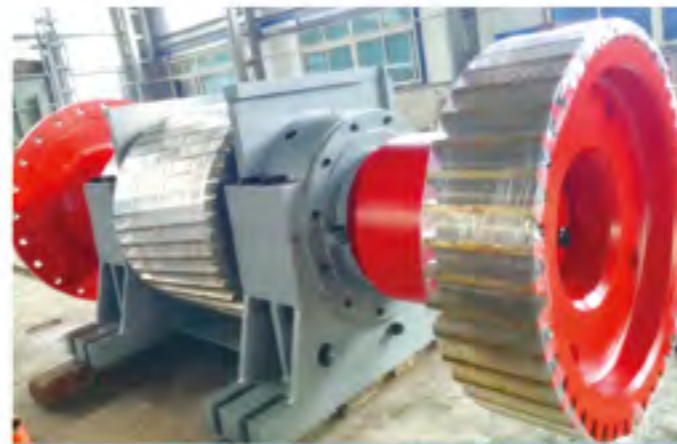
球磨机驱动齿轮/ Drive Gear of Ball Mill
